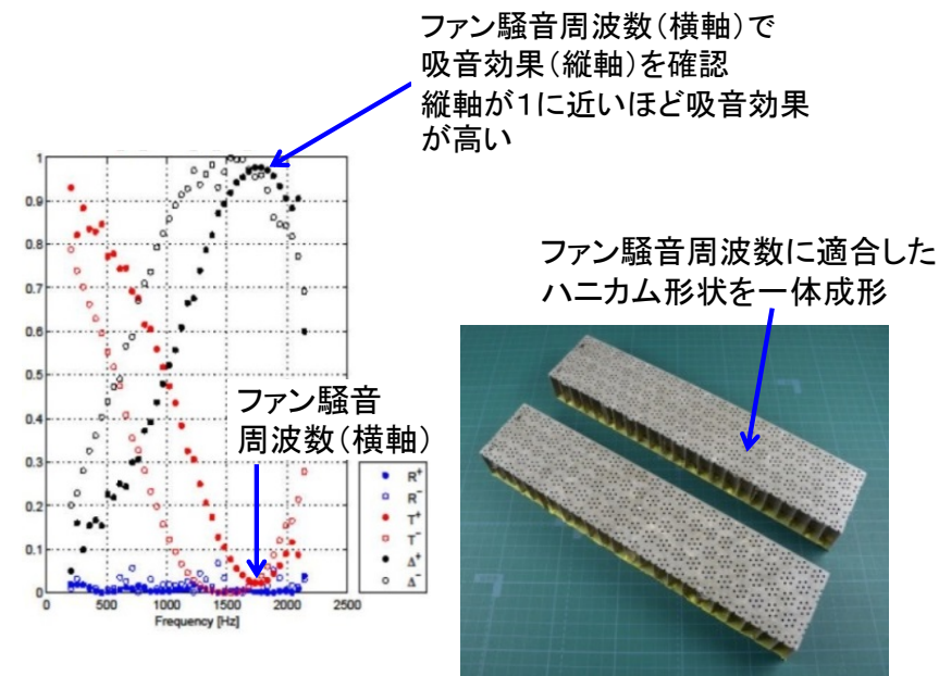
樹脂製ライナパネル供試体と吸音特性
