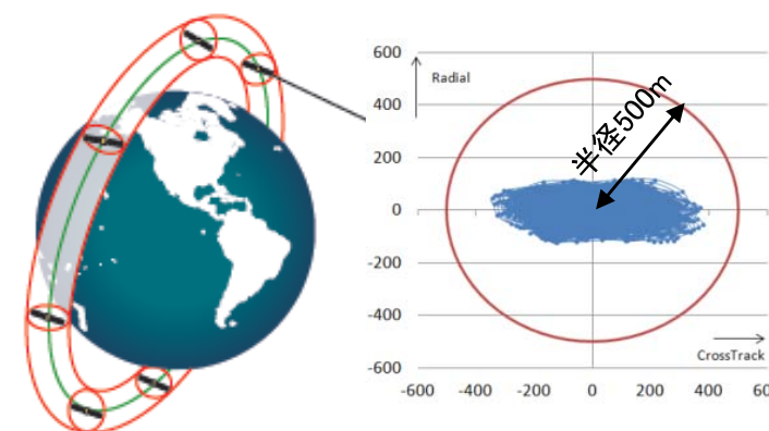
自律軌道制御による軌道保持
