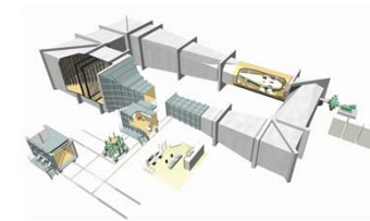
2m×2m低速風洞
