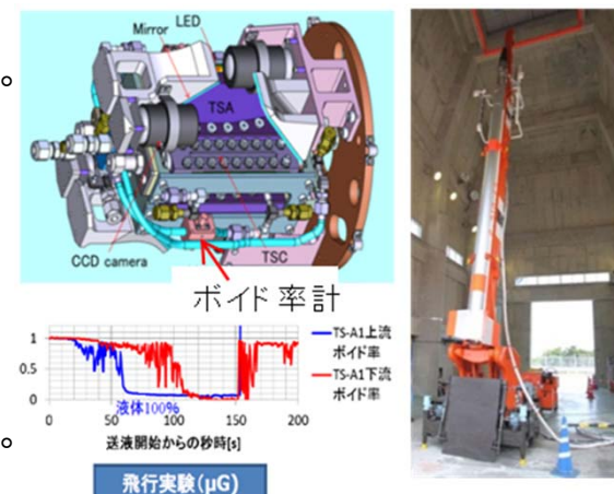
観測ロケットS-310-43におけるボイド率計測
