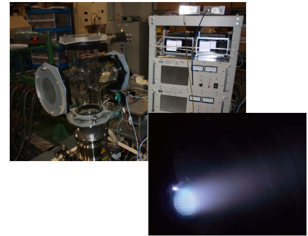
イオンエンジン中和器の耐久試験 (⑦)
