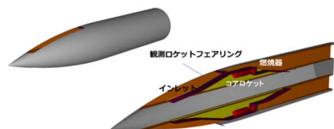
極超音速の試験形態案
