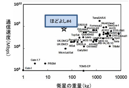
近地球衛星の重量と通信速度 (⑧)
