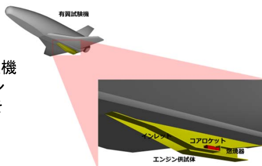
超音速の試験形態案
