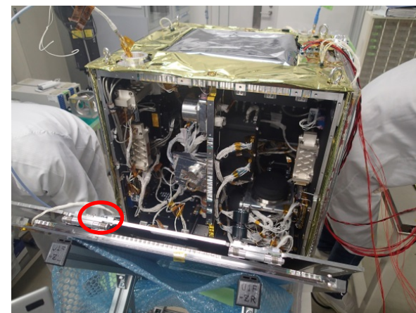
PROCYON内部に搭載されたGaN SSPA
