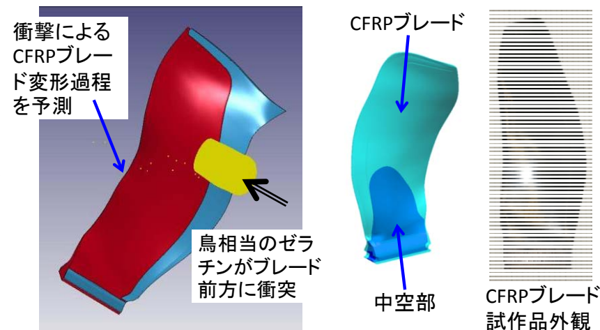
CFRPブレード衝撃解析結果、中空CFRPブレード試験供試体
