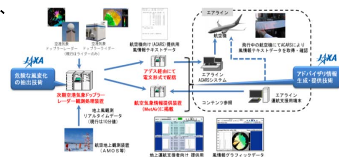
気象庁によるALWINの運用形態とDREAMS技術の適用部分
