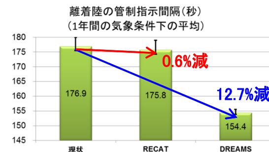
羽田空港(南風運用)での間隔短縮効果比較
