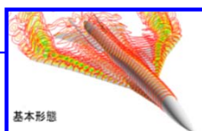
小型SSTの低速性能解析結果
