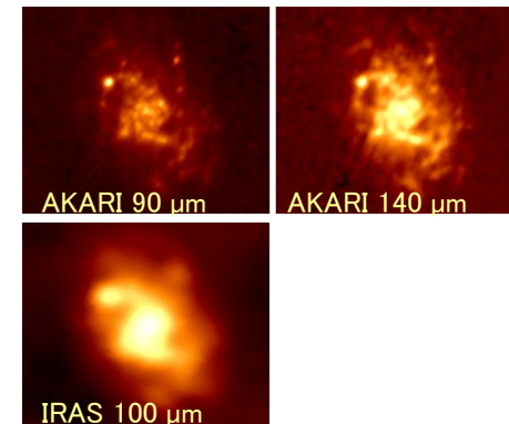
渦巻き銀河の遠赤外線画像の比較。 1983年に米英蘭が行った観測に比べ、「あかり」は解像度が数倍改善しているほか、より長波長での情報が得られている。(①)
