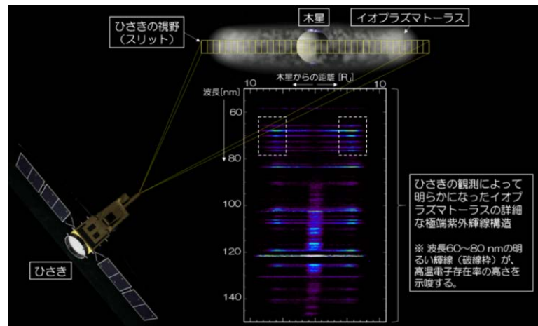
SPRINT-A (ひさき) が観測したイオプラズマトーラスの極端紫外スペクトル
