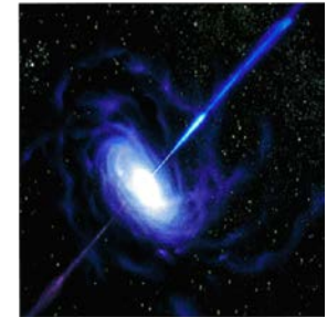
ジェットを放出する 巨大ブラックホール Mkn421のイメージ
