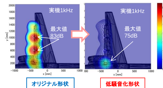
低騒音フラップの騒音計測結果
