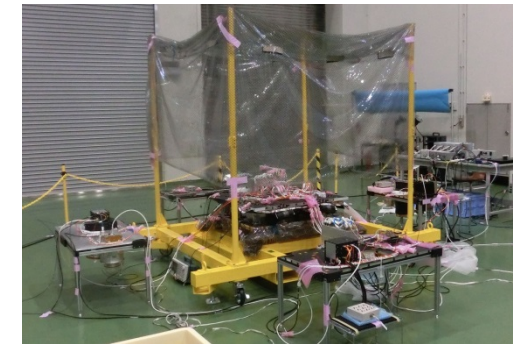
ミッション部総合試験の様子
