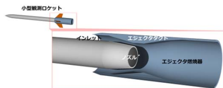
遷音速の試験形態案
