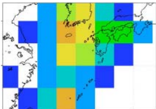
CMAP (NOAA)
