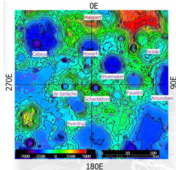
左：ISECG等で使用された月極域の詳細地形データ。 南極点を中心とする300km四方の領域。 色は標高を表す。
