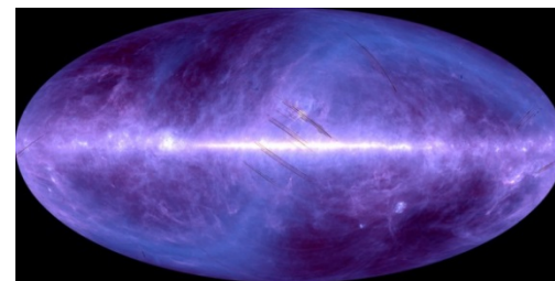
遠赤外線で見えた全天の様子 中央横に明るい帯が天の川
