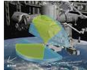
MAXIでX線変動を 長期間観測
