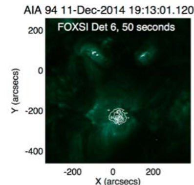
FOXSI-2で得た硬X線画像 (②)
