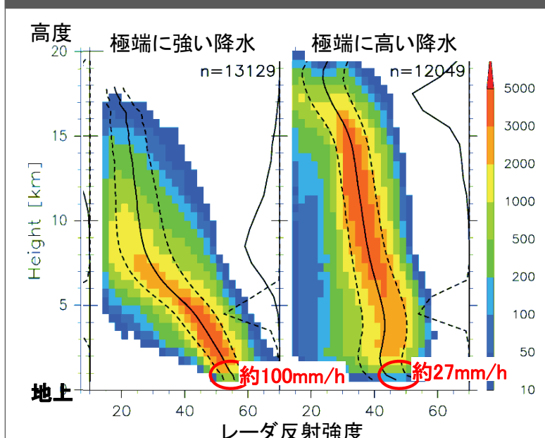
TRMM観測域の陸上における、各2.5度格子での上位0.1%の強い地表降水vs 高い降水イベントの鉛直構造
