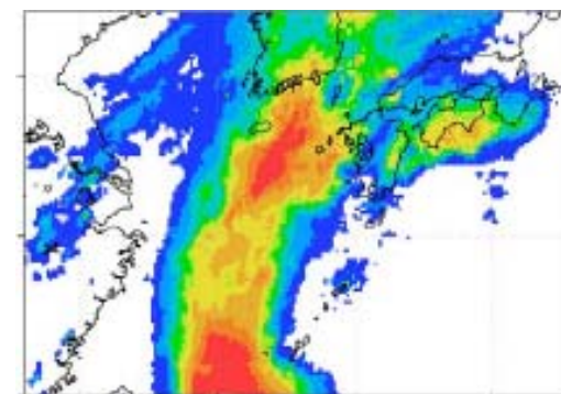
GSMaP (JAXA)
