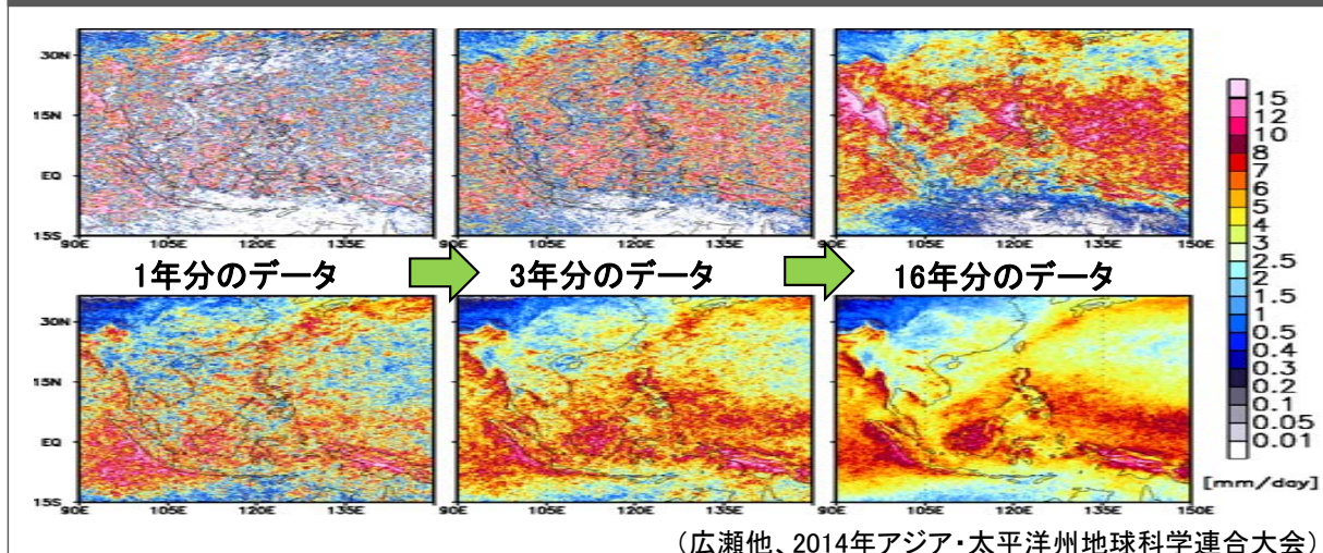
蓄積年数別の8月平均(上)および年平均(下)の降水分布
