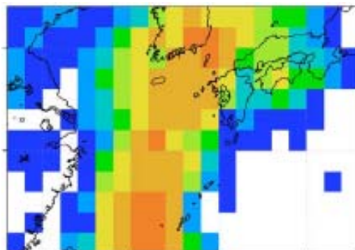
GPCP-1DD (NASA)
