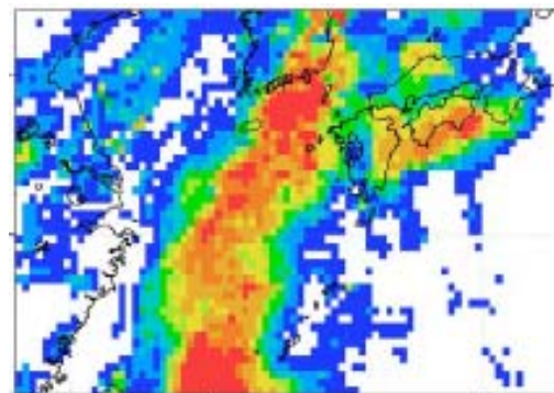
TMPA 3B42 (NASA)
