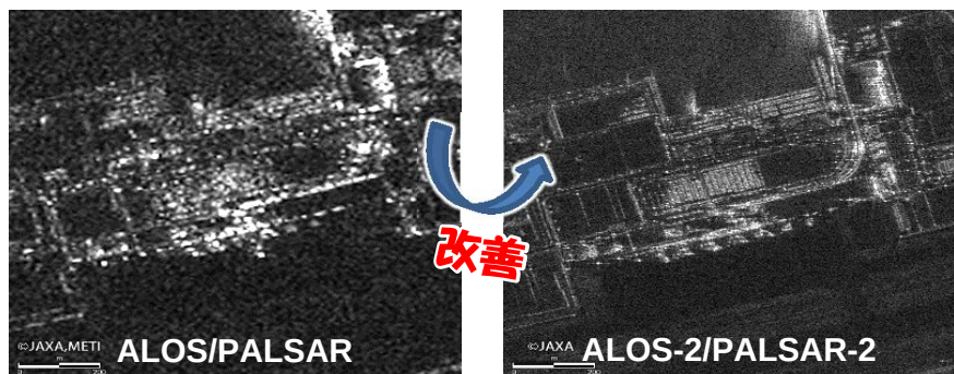
ALOSとALOS-2の画像との比較
