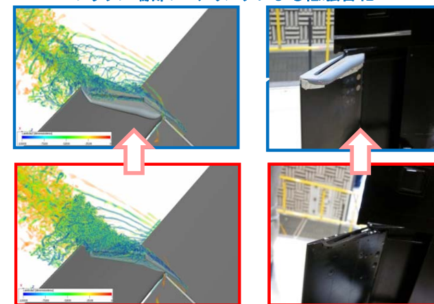
オリジナルのフラップ端部形状
