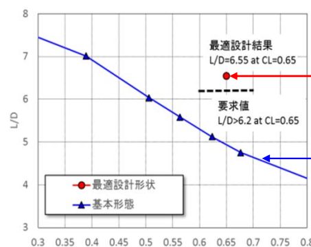
小型SSTの低速性能解析結果
