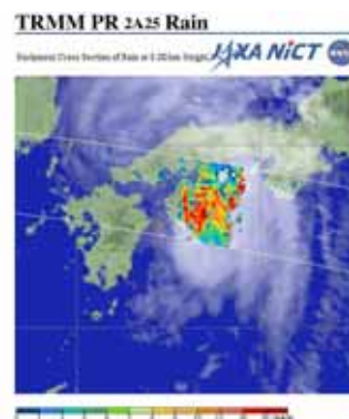
台風10号の降雨分布と雲画像
