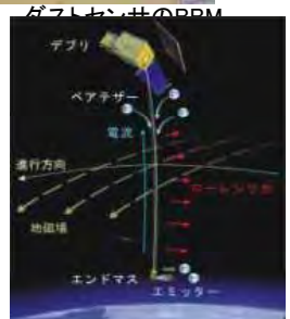
導電性テザーによるデブリ除去ミッション
