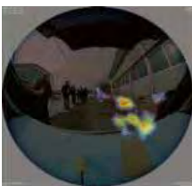
宇宙観測用*に開発した軟ガンマ線観測装置を応用した放射性物質分布可視化装置「超広角コンプトンカメラ」の実証実験結果(2012年3月29日報道発表) *ASTRO-Hに搭載予定
