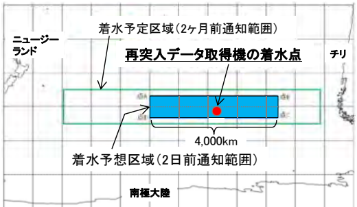
着水予想区域と再突入データ取得機の着水点
