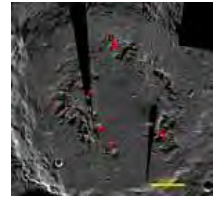
南極エイトケン盆地シュレーディングークレータでかんらん石が同定された(赤丸)
