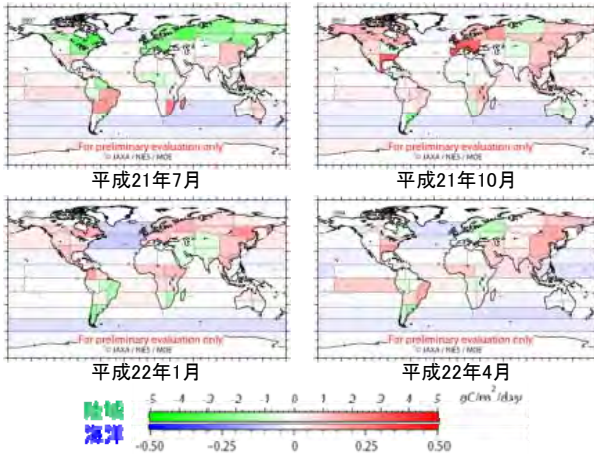
GOSAT及び地上観測データによる二酸化炭素ネット吸収排出量分布
