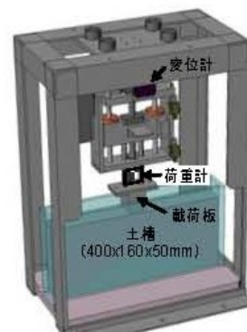
(a) 載荷装置のCADイメージ
