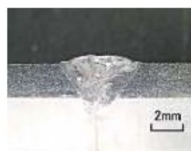
(b) 溶接部マクロ組織
