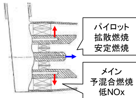
(図3) ステージング燃料ノズル
