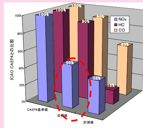
Rich-Lean燃焼方式 環状燃焼器
