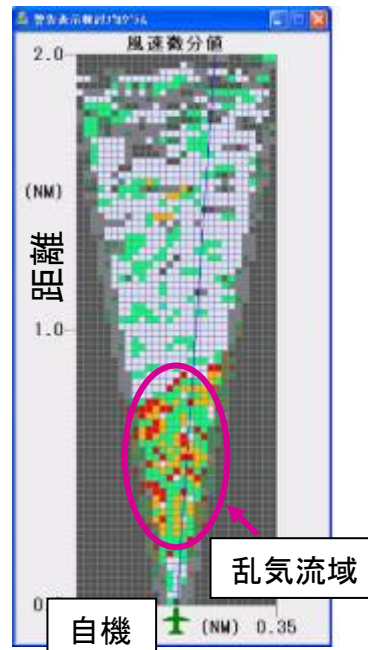
試作中のコックピット表示画面
