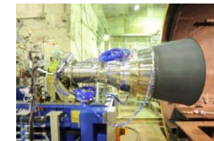
高空燃焼試験 (JAXA角田)
