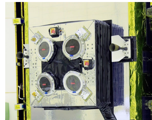
はやぶさ2イオンエンジン (© JAXA)
