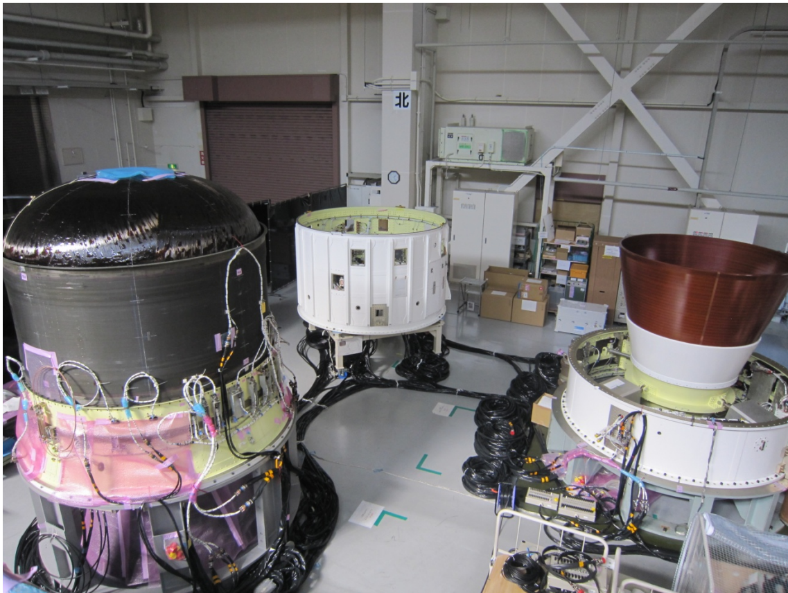
イプシロンロケット試験機のシステムチェックアウト試験の様子
