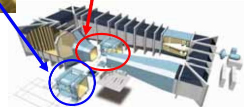
6.5m×5.5m低速風洞
