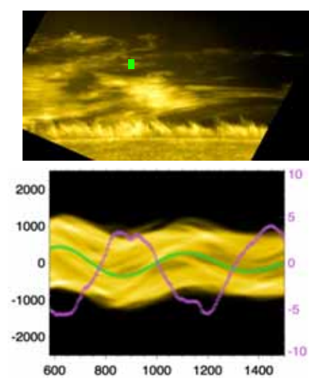
緑色の領域のプロミネンス震動を、「ひので」とIRISで同時観測し、波動散逸を同定した。
