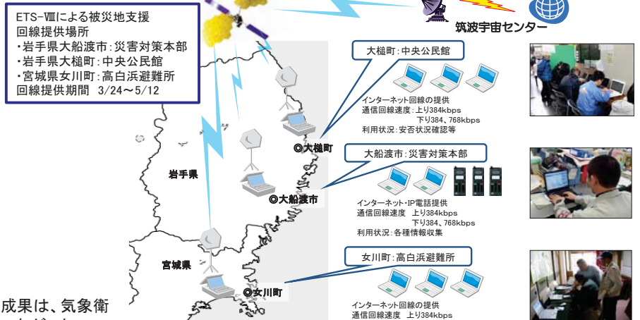
東日本大震災支援におけるETS-VIII通信概念図
