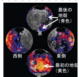
「かぐや」の観測データによる研究により得られた月地殻の形成過程 色は地殻が形成された時期の違いを表し、黄色が最も古く、橙・赤・青への新しくなる。月の裏側中央の黄色の領域で最初に地殻が誕生し、周囲、そして月の表側へ徐々に地殻が広がったことが明らかにされた。
