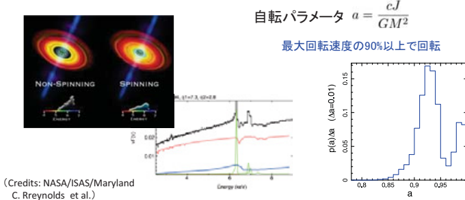
鉄輝線による活動銀河核の巨大ブラックホール自転への制限
