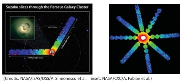
銀河団の外縁 (= 宇宙の大構造進化の現場) からのX線放射
