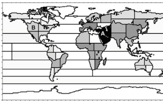
GOSATデータを取り込んだことによる二酸化炭素吸収排出量推定誤差の低減率(年平均)
