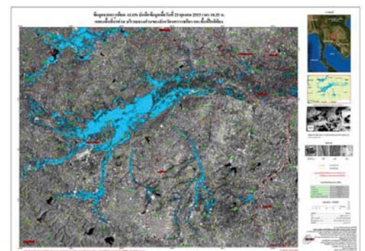
平成22年10月タイ洪水の浸水域図
