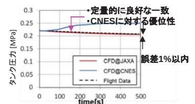
図2. タンク内圧力履歴の比較
