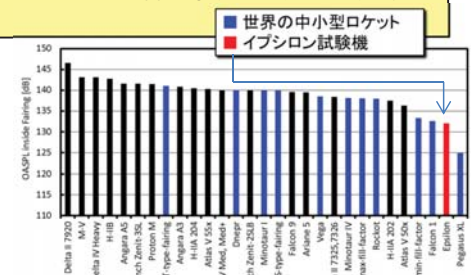
図1. 他のロケットとの音響レベルの比較
