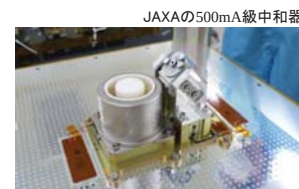
JAXAの500mA級中和器
