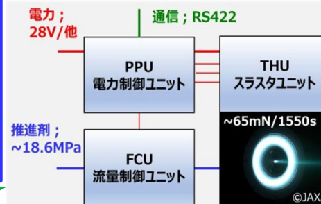
小型ホールスラストの構成
