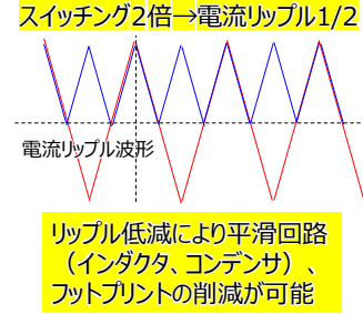
高速スイッチング、及び平滑回路削減の説明図
