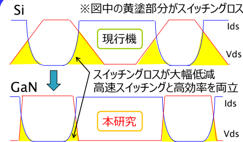
高速スイッチング、及び平滑回路削減の説明図
