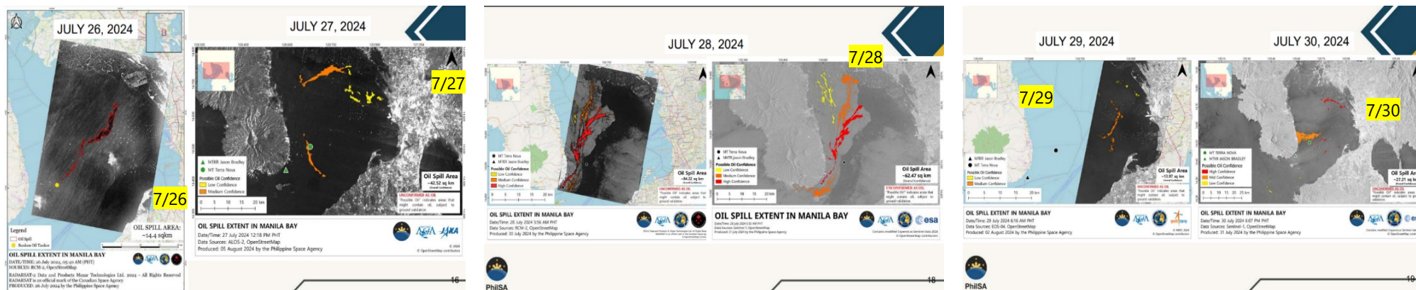
マニラ湾で発生したタンカー沈没海難に伴う油流出事故に関する各日ごと油漂流解析図（7/26～7/30）
