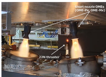
地上システム燃焼試験例 (SLIM)
