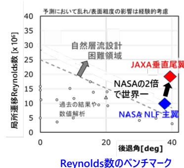
Reynolds数のベンチマーク
