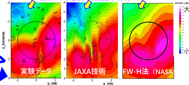
図5: 機体下方位置での騒音推定結果ベンチマーク
