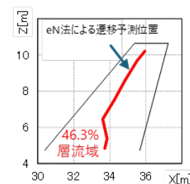
実機で予測される遷移位置(滑面)
