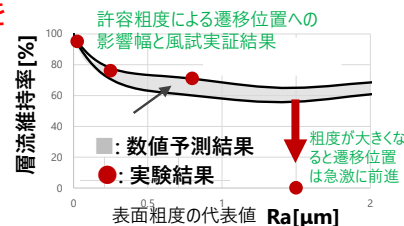
粗度による層流化効果への影響確認
