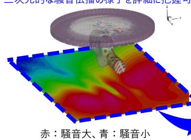
図4: ヘリ形状の騒音伝播解析 三次元的な騒音伝播の様子を詳細に把握可能
