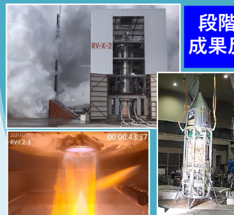
RV-Xの組み立て、落下試験、燃焼試験
