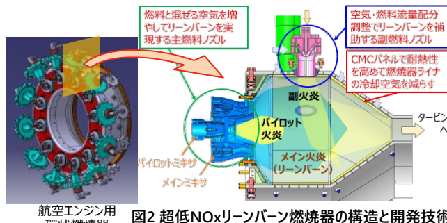
図2 超低NOxリーンバーン燃焼器の構造と開発技術
