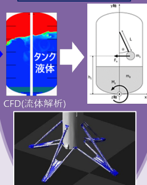
CALLISTO のシステム設計
