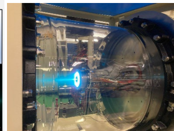
THUの試験の様子
