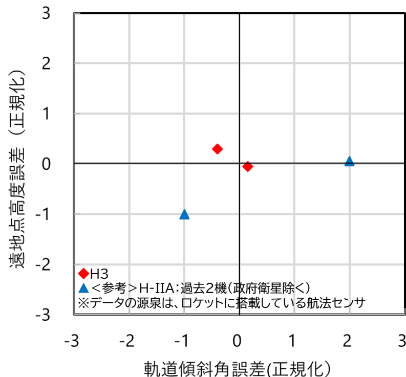
静止トランスファー軌道等の軌道投入精度 (H-IIAロケット44号機のデータで正規化)
