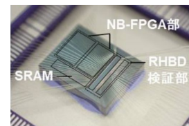
16nm FinFET NB-FPGA 300mmウェハ、テストチップ外観
