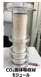
図3 CO 2 分離濃縮装置 © 株式会社JCCL
