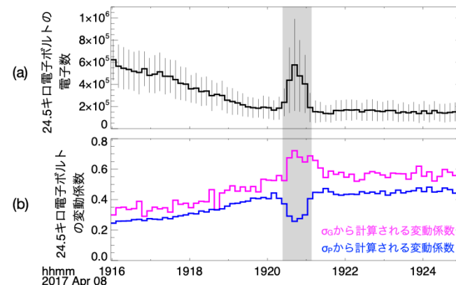
コーラスによる電子の超高速加速の痕跡を「あらせ」衛星の観測により発見
