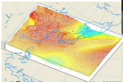
可降水量推定による気象数値予報初期値同化
