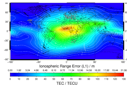
宇宙天気予報（全電子数マップ）
