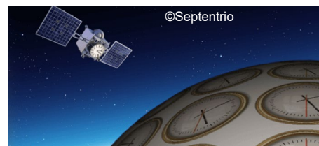
地球物理科学への応用・貢献
