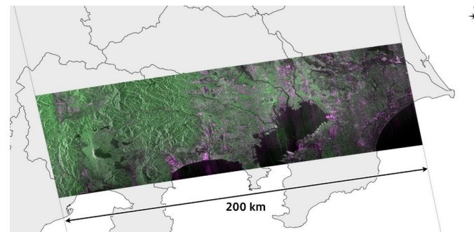
「だいち4号」PALSAR-3による関東の初観測画像 (観測幅：200 km)
