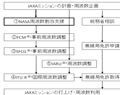
図 国際周波数調整・無線局免許取得の主な流れ※1
