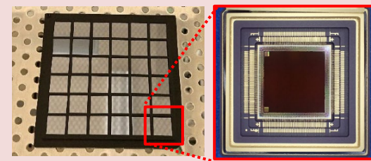
ダイシング後チップ（左）と開発された次世代MPU（右）
