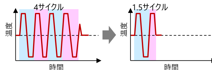
システム熱真空試験の温度プロフィール
