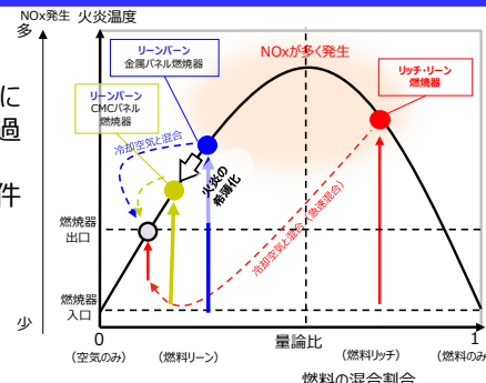
図1 NOx発生メカニズムとリーンバーンの必要性
