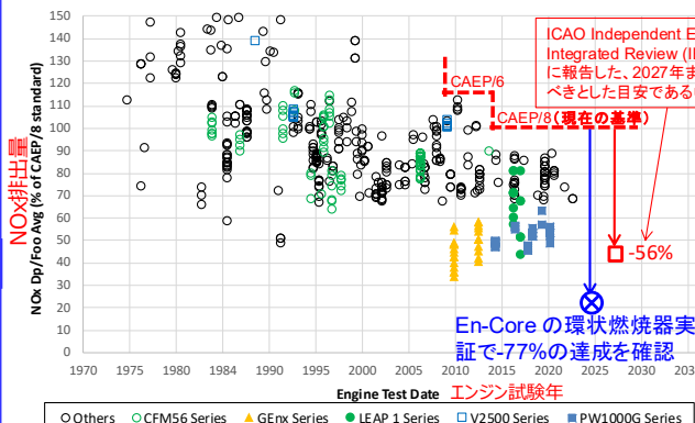
図3 ICAO Emission Data Bank Issue 30 (23 July 2024)に基づくベンチマーク
