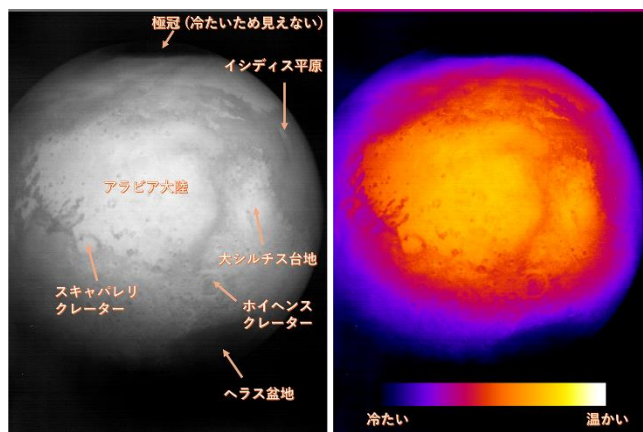
↑TIRIが約4万kmの距離から撮像した火星。TIRIの検出限界以下の低温の極冠や、太陽系最大規模の衝突クレータであるヘラス盆地が低温領域として確認できる。（左）輝度温度画像、（右）高温を暖色で表示した画像。（クレジット：ESA/JAXA）
