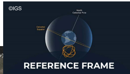
国際基準座標系生成への貢献
