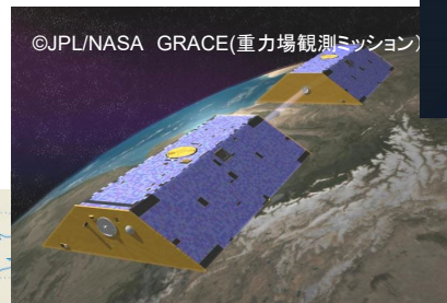
地球物理科学への応用・貢献
