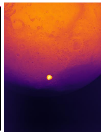
↑TIRIが約1000kmの距離から撮像した衛星Deimosの画像。（上）連続画像（下）高温を暖色で表示した画像。（クレジット：ESA/JAXA）
