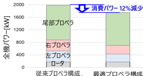
図3 前進飛行時の全機パワーの比較
