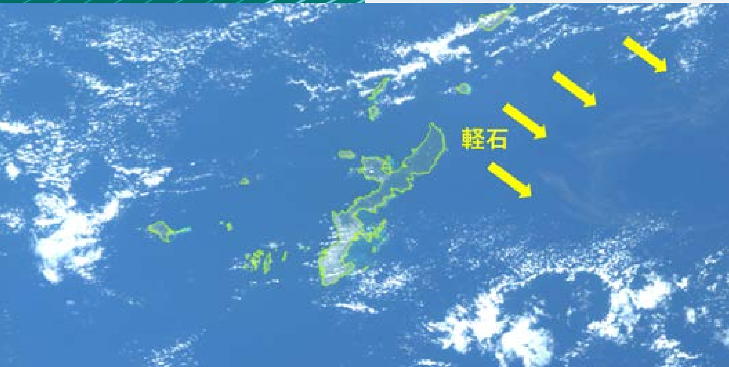
写真：気候変動観測衛星「しきさい」(GCOM-C)が捉えた 福島第一原子力発電所の噴火により発生した軽石漂流の様子
