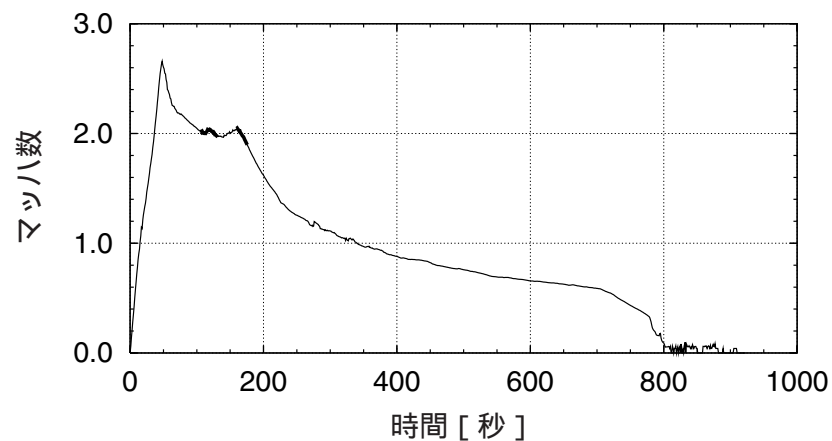
図3：飛行速度の時間変化
