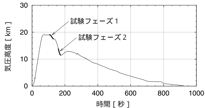
図2：飛行高度の時間変化
