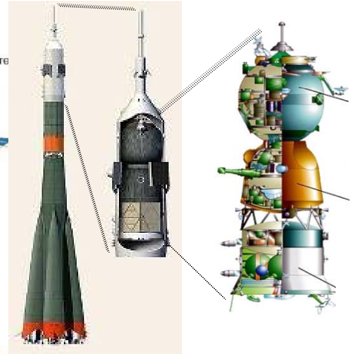
ソユーズロケットと宇宙船
