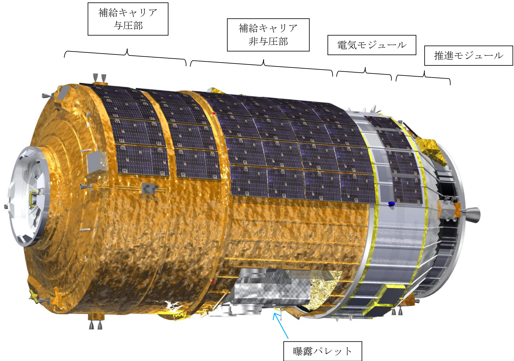
図-7 「こうのとり」6号機 外観図
