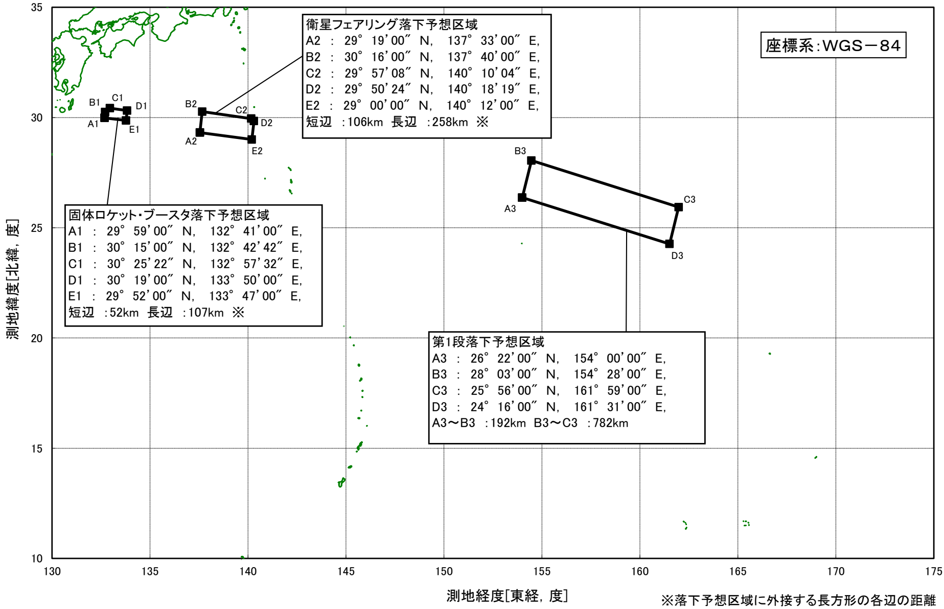
図-11 ロケット落下物の落下予想区域
