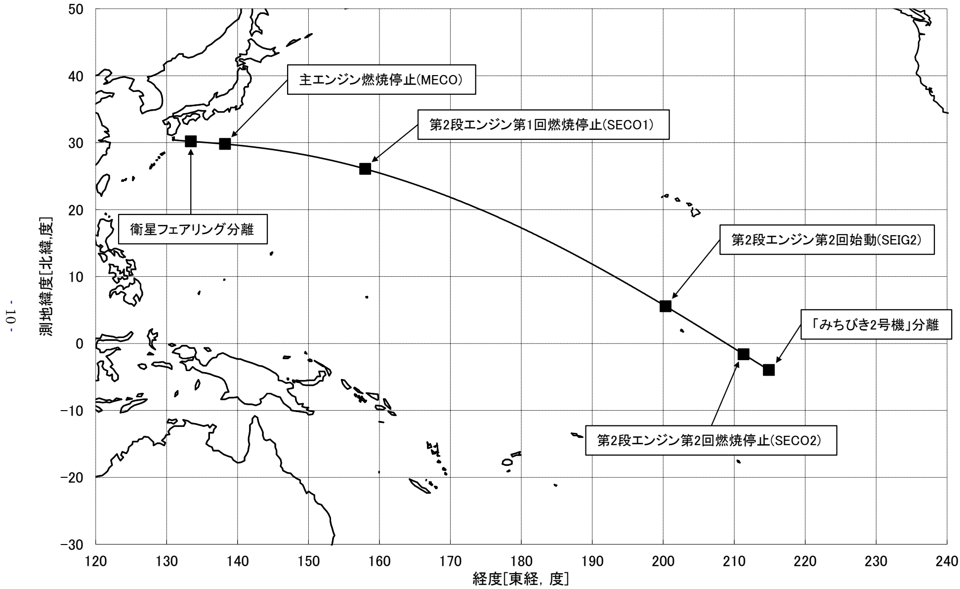
図-5 ロケットの飛行経路
