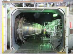
LE-5B-3認定型エンジン燃焼試験 (左: MHI田代試験場、右: 角田宇宙センター)
