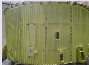
実機大工作・強度試験 (MHI大江工場)
