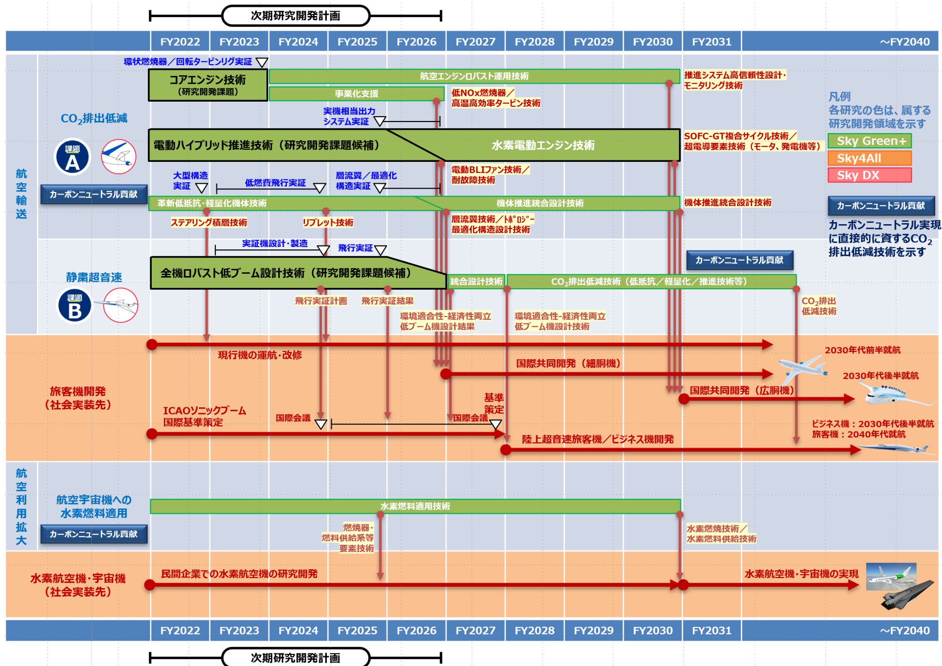
図4.3.2 カーボンニュートラルの実現に資する研究開発ロードマップ案
