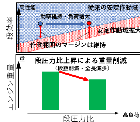
図2 圧縮機安定作動領域拡大効果
