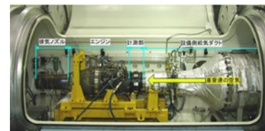
水素エンジン実環境試験設備 (高気性能試験設備の水素対応化)
