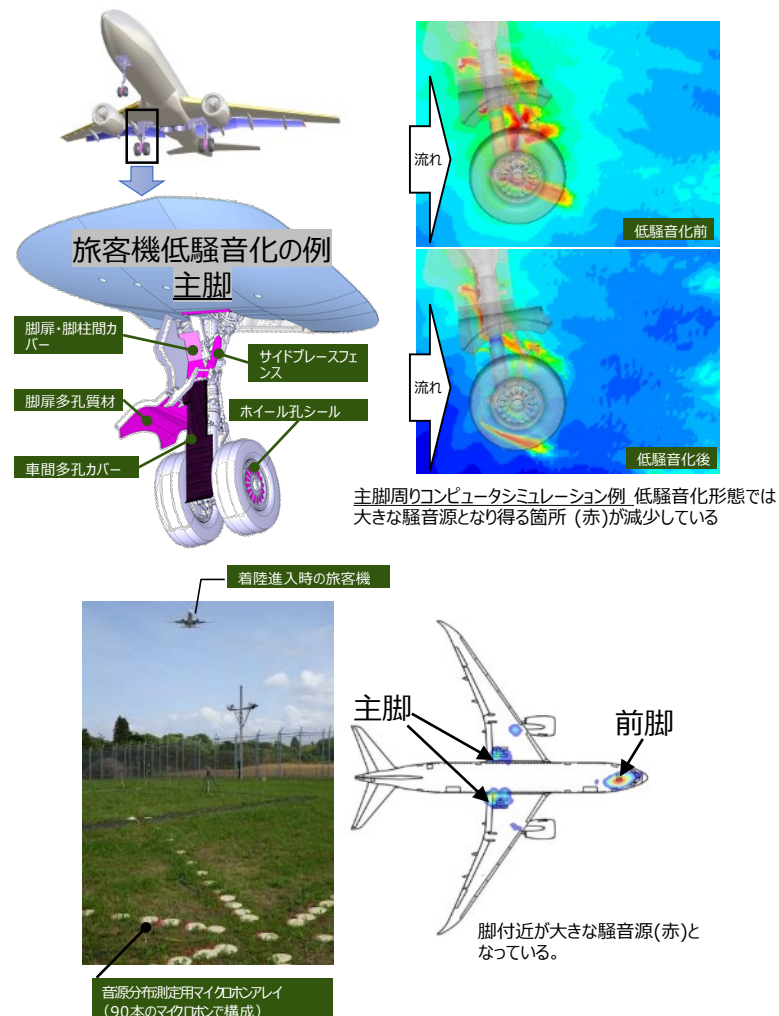
着陸進入時の旅客機の飛行音源探査結果例 測定の様子(左図)と実測結果(右図)
