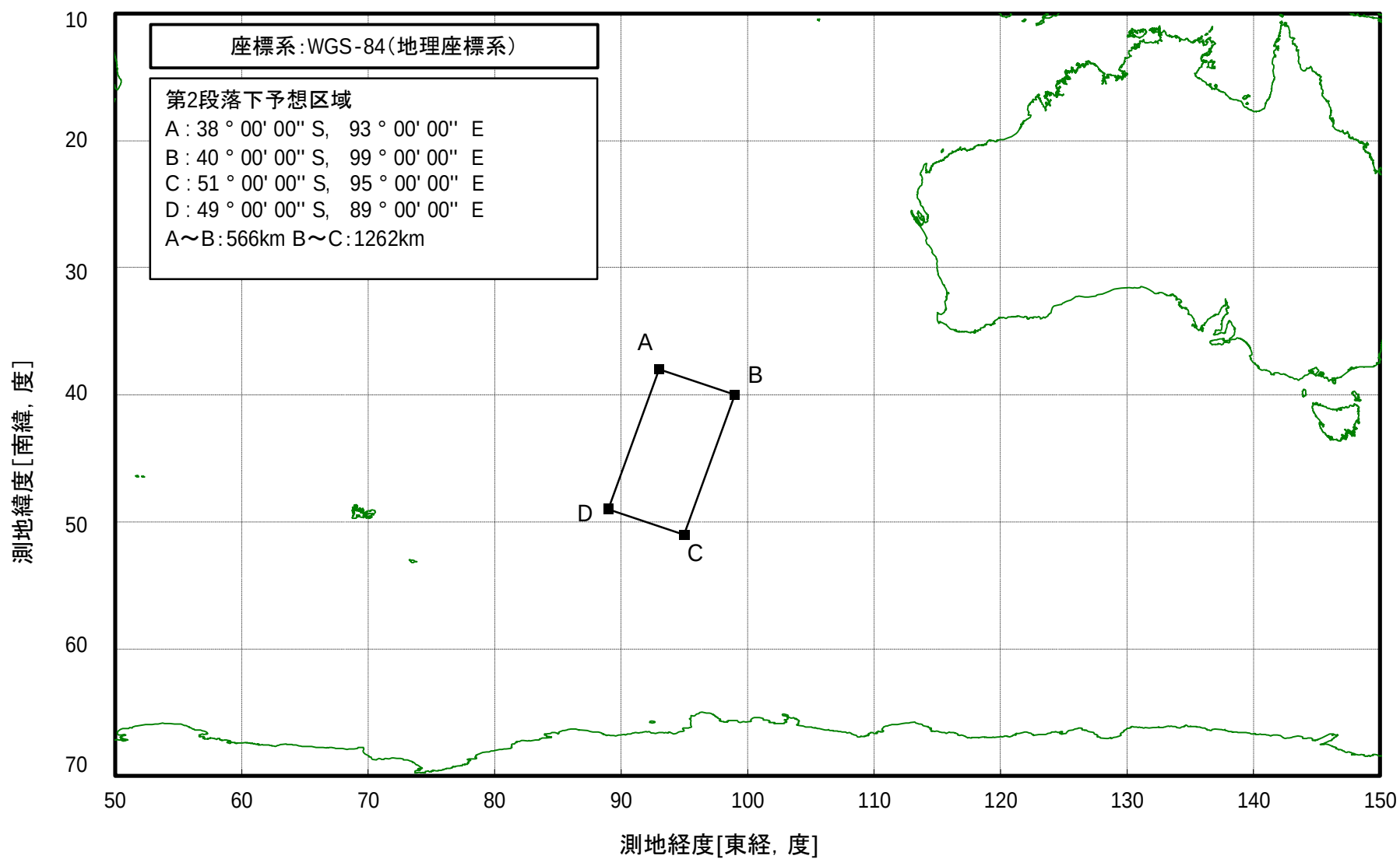
図-11 第2段階ロケットの落下予想区域
