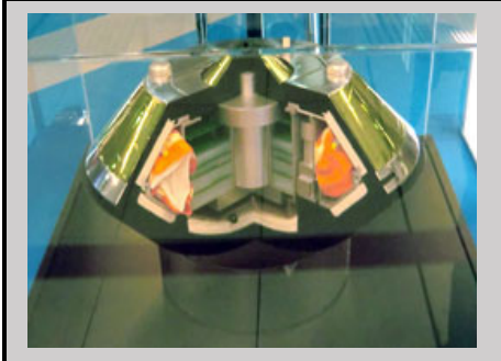
HP-0238-01 「はやぶさ」回収カプセル模型(カットモデル)
