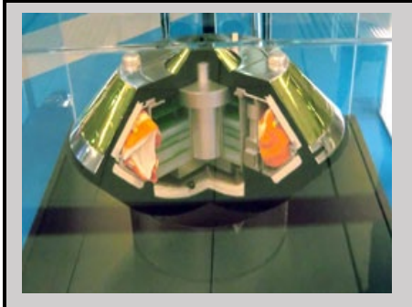
HP-0238-01 「はやぶさ」回収カプセル模型(カットモデル)
