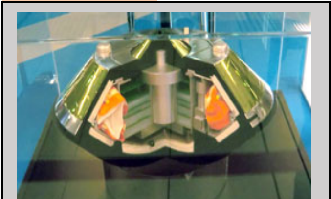
HP-0238-01 「はやぶさ」回収カプセル実物大模型（カットモデル）
