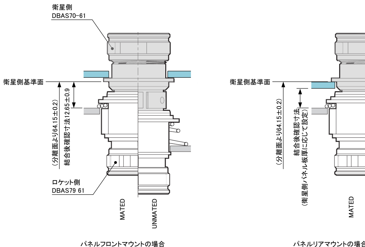
図 A3-5 分離コネクタ位置と位置誤差(高さ方向)及び結合後寸法計測位置
