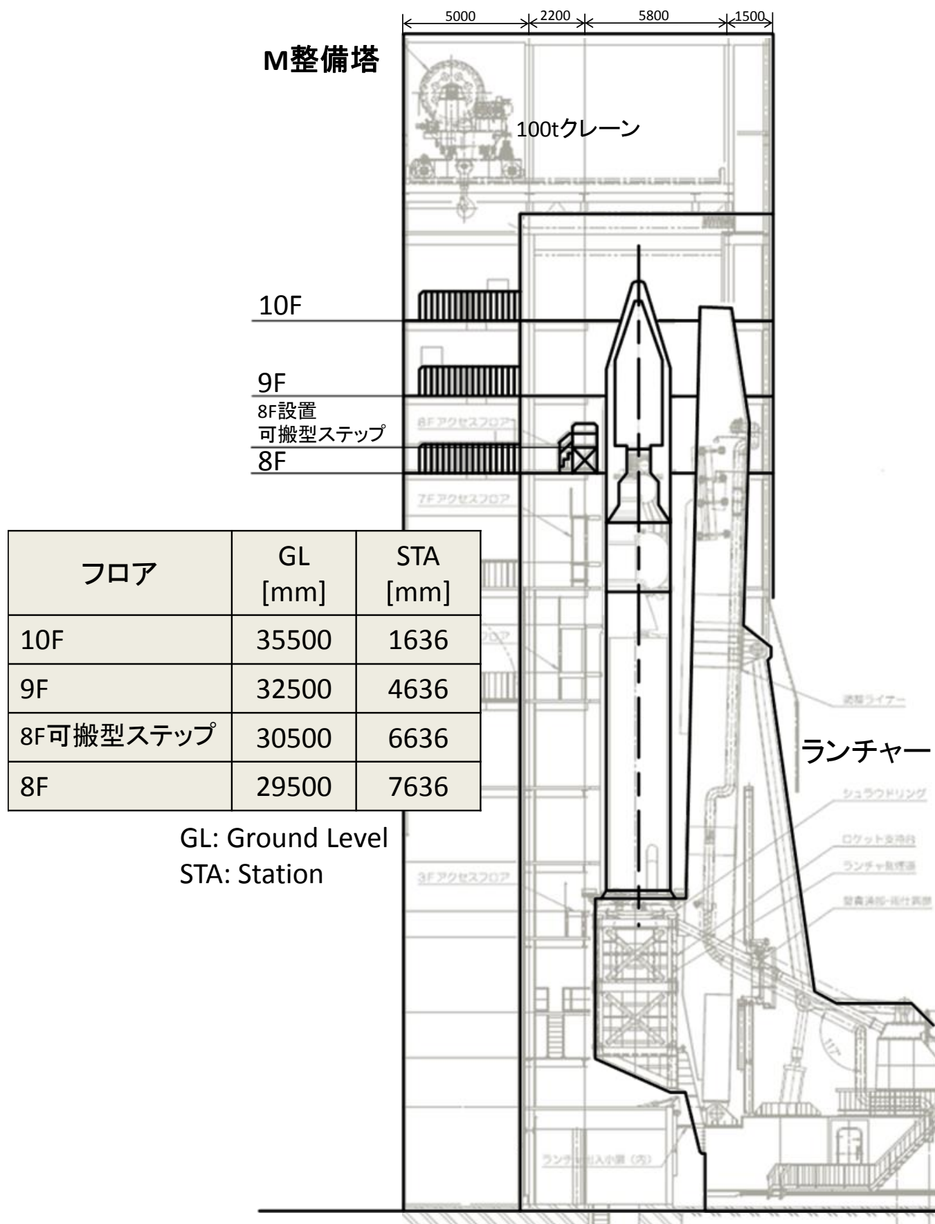
図 D1-1 M 整備塔フロア高さ
