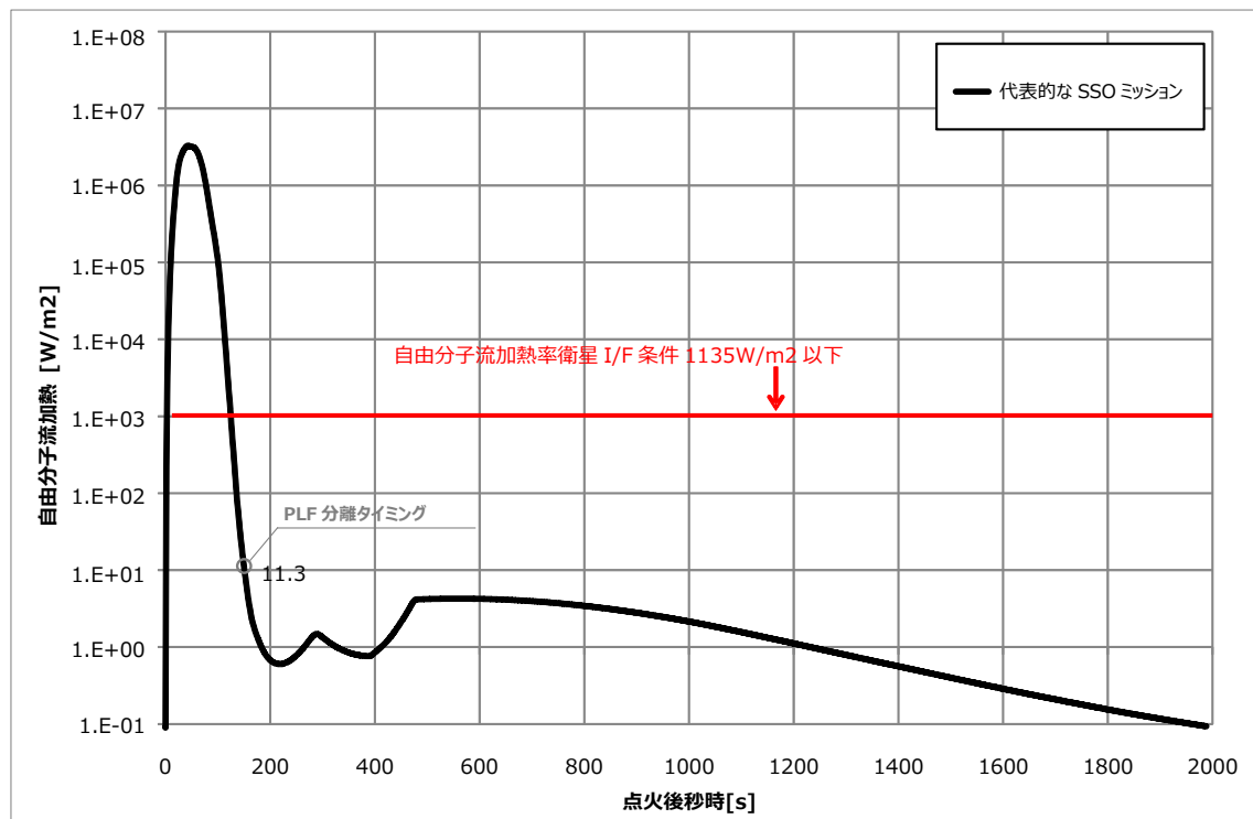
図 4.5.2-3 ロケットの自由分子流加熱率履歴(ノミナル軌道)
