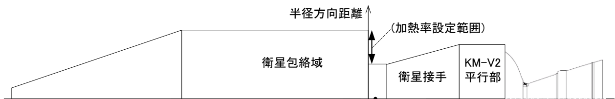
図 4.5.2-4 3 段モータブルーム輻射加熱率条件
