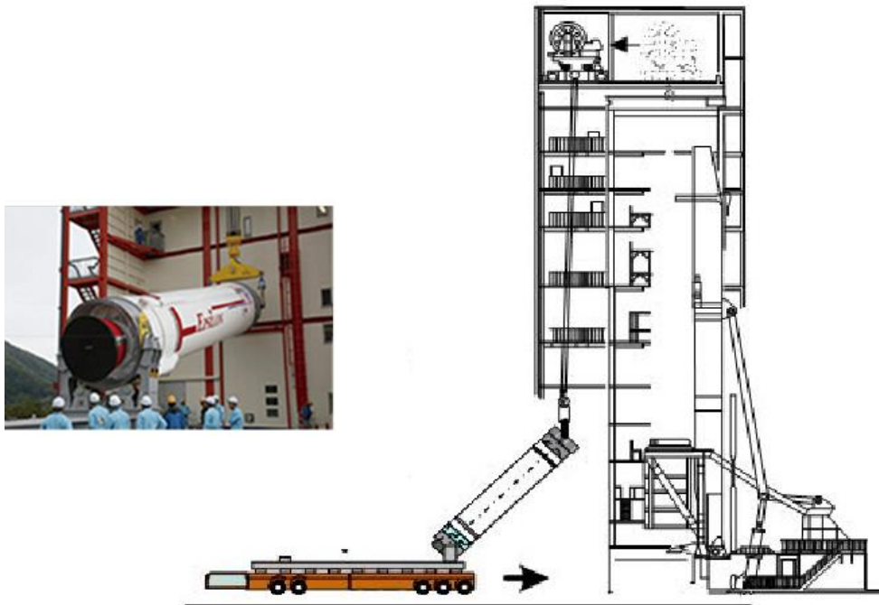
図 6.4-7 1段機体搭載
