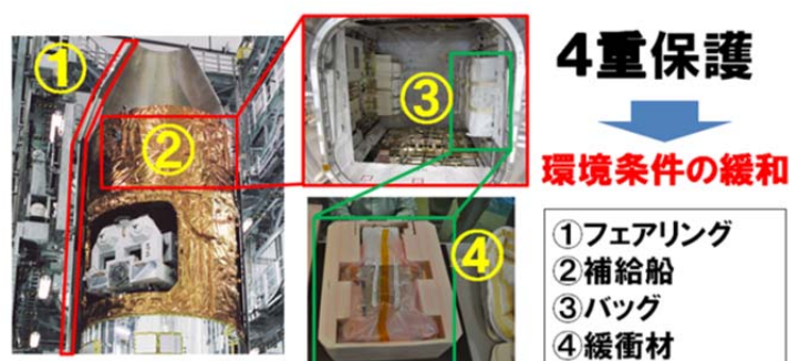
図 5.1.3-3 「こうのとり」で超小型衛星を打ち上げる際の環境
