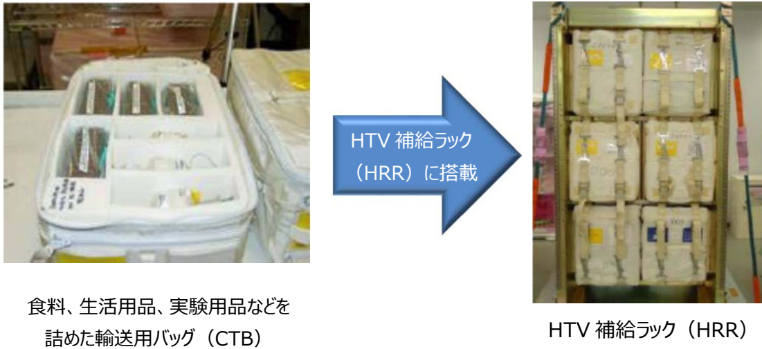
図 5.1-3 船内物資の搭載例 (JAXA)
