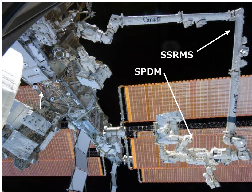
SPDM「デクスター」を使って米国の船外物資を運搬する様子（NASA） （HTV2で運搬したFHRの移動）
