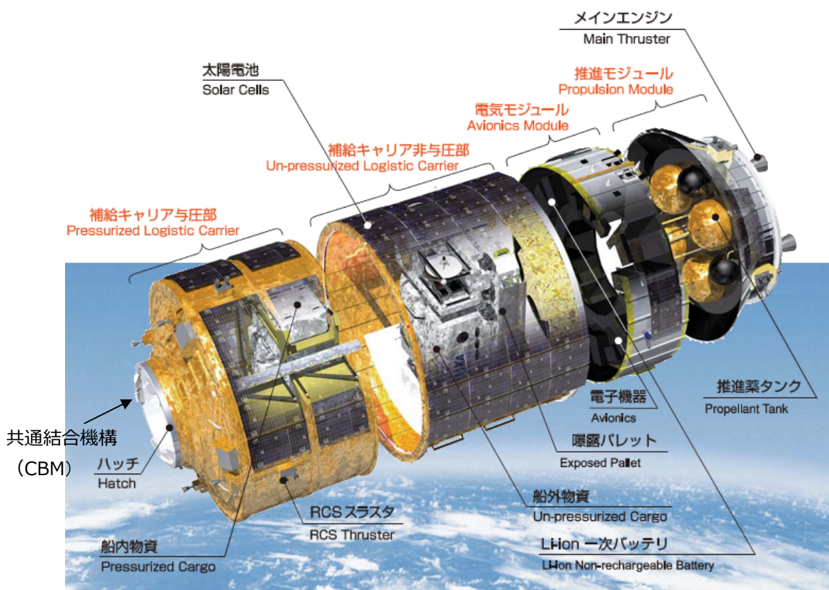
図A1-1 「こうのとり」の全体構成（JAXA）
