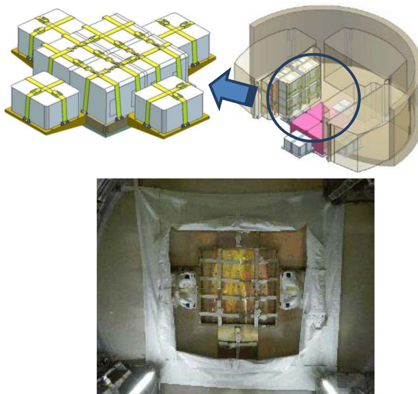
図 5.1-4 5号機から新設した HRR の搭載構造 (JAXA)
